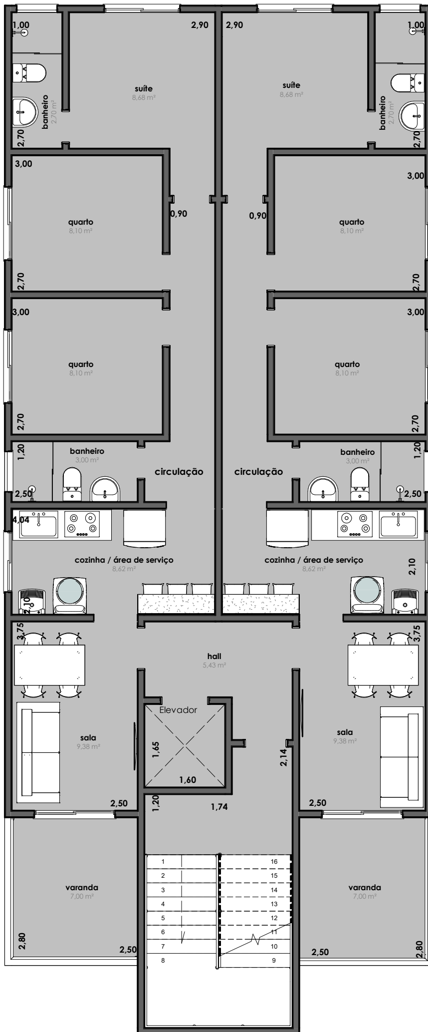
PAVIMENTO TIPO - RESIDENCIAL ALDAIR SOUZA
